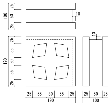
HB-4**H 空洞レガ 4 ツ穴 菱形 190×190×100・120・150
